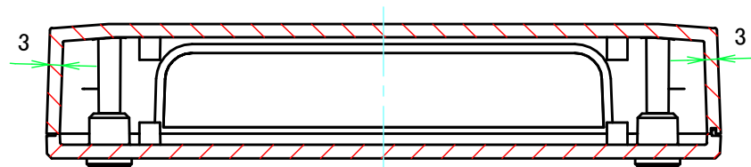
B-B ( 1 : 1.5 )
